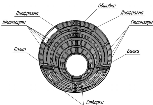
Рис. 2. Схема отсека ВСУ (вид против полета)
