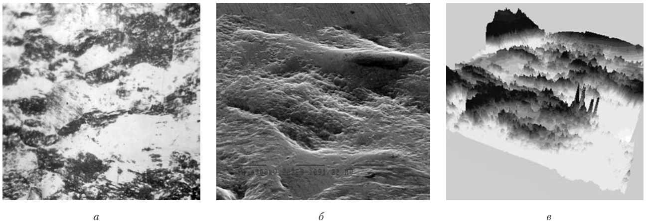
Рис. 1. Изображения деформационного рельефа поверхности лакированного алюминиевого сплава Д16АТ, полученные различными методами регистрации: оптическая микроскопия \times 300 (а); электронная микроскопия \times 5000 (б); бесконтактная интерференционная профилометрия (в)
