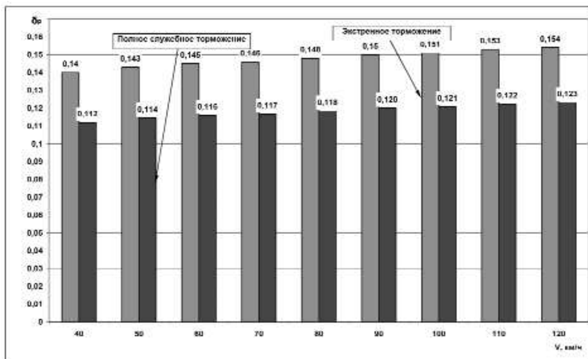
Рис. 2. Расчетные коэффициенты сил нажатия тормозных колодок
