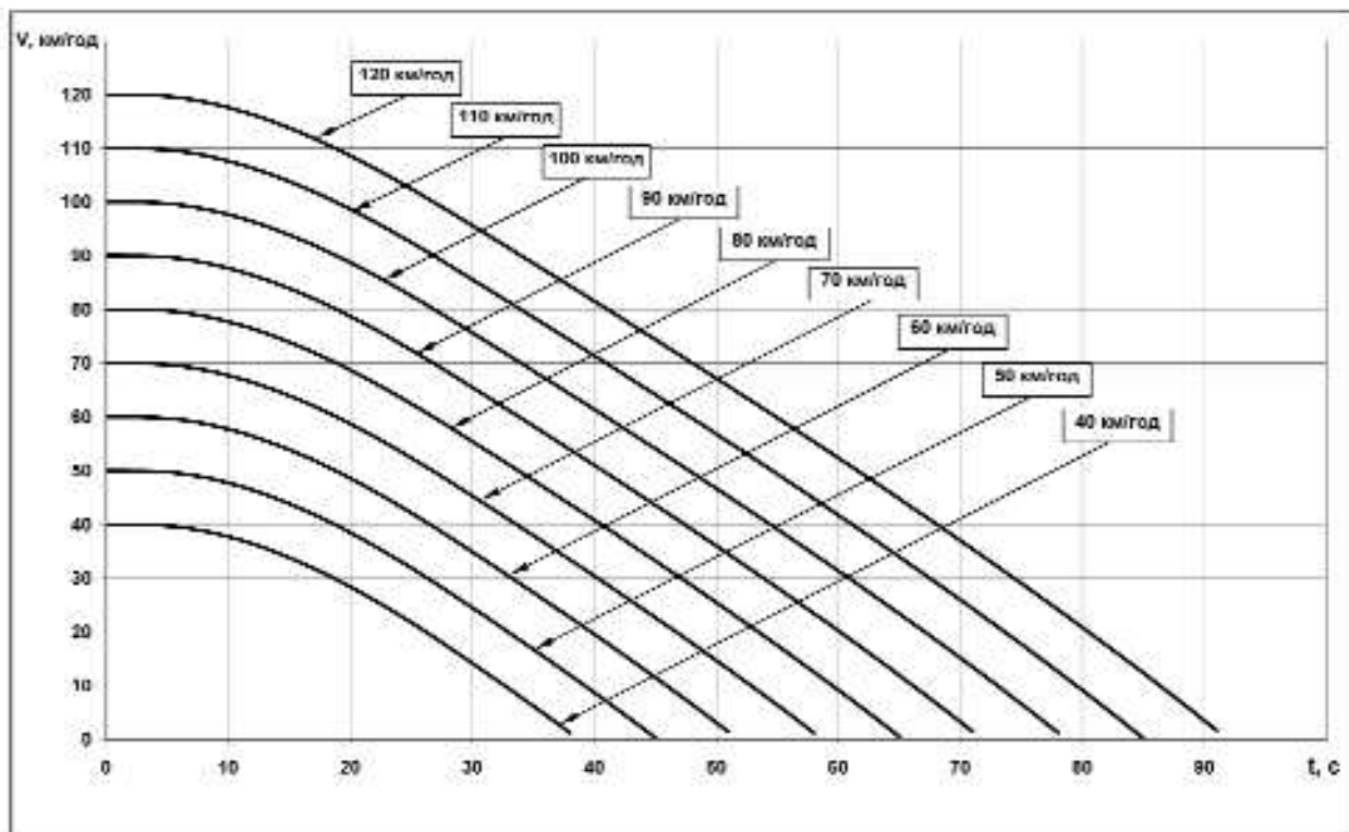
Рис. 6. Изменение скорости движения вагона при торможении
