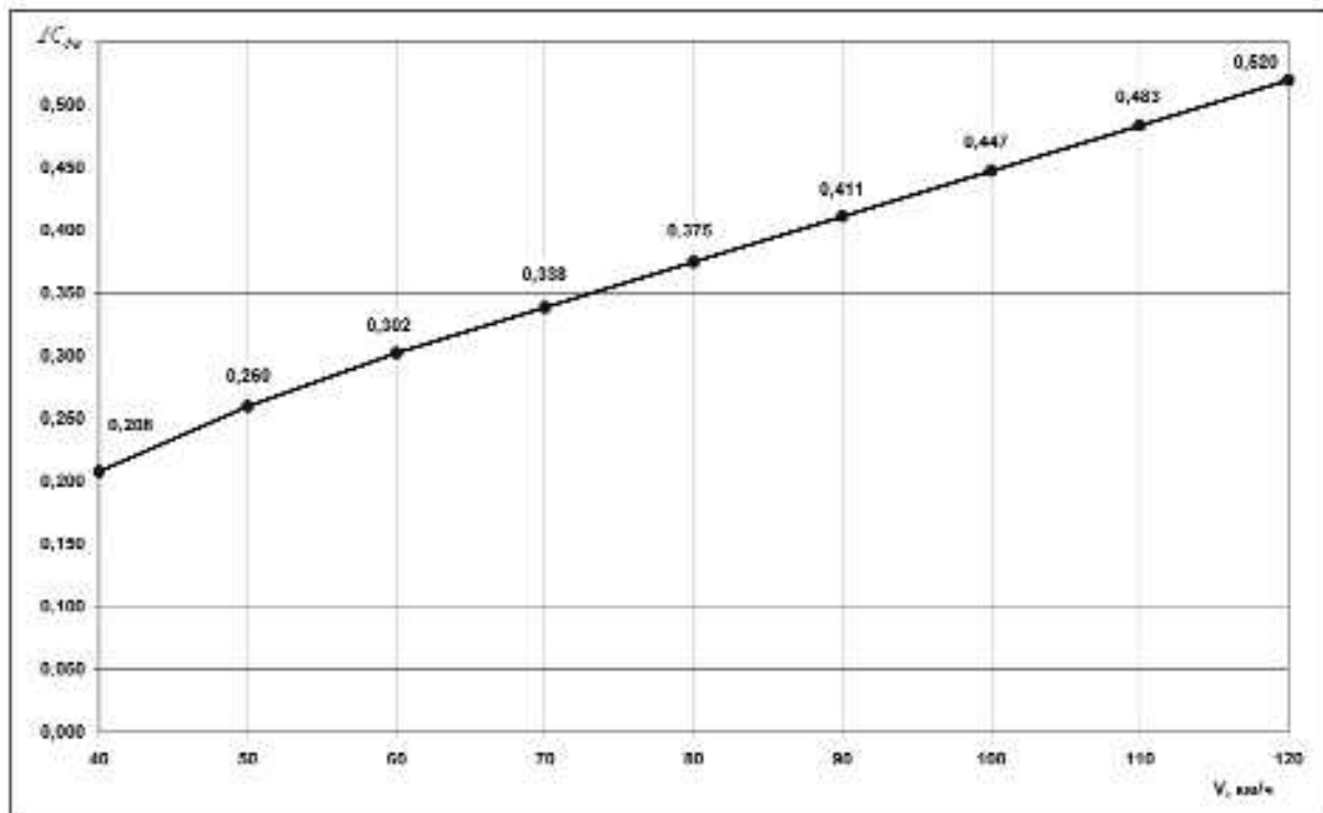
Рис. 5. Коэффициенты вертикальной динамики необрессоренных частей тележек
