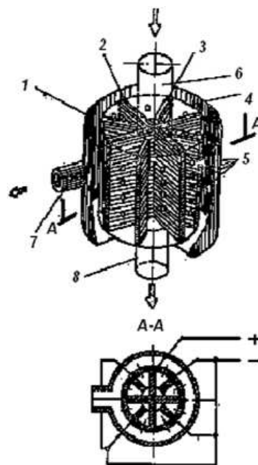
Рис. 1. Принципова схема робочої комірки електросепаратора
