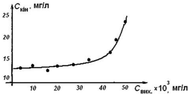
Рис. 4. Залежність очистки палива ТС-1 від початкової концентрації забруднення ( C_{\text{кін}} – кінцева, C_{\text{вих}} – вихідна)
