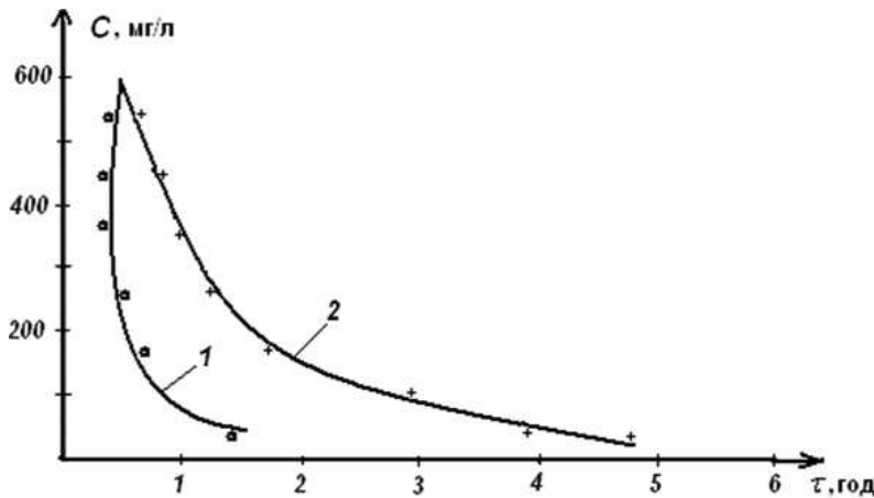
Рис. 5. Вплив часу сепарації на очистку нафтопродуктів: 1 – паливо ТС-1; 2 – масло АМГ-10
