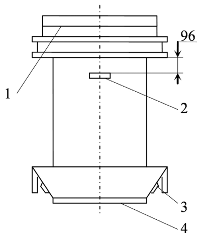
Рис. 5. Место размещения заряда в верхнем баке трансформатора: 1 – уровень масла; 2 – заряд; 3 – разгрузочные клапана; 4 – заглушка
