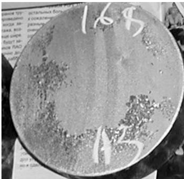
Рис. 2. Макроструктура поковки жаропрочного сплава ХН77ТЮР-ВД, содержащего 20,13% хрома, 75,09% никеля, 0,91% алюминия, 2,74% титана, 0,06% углерода, 0,38% железа
