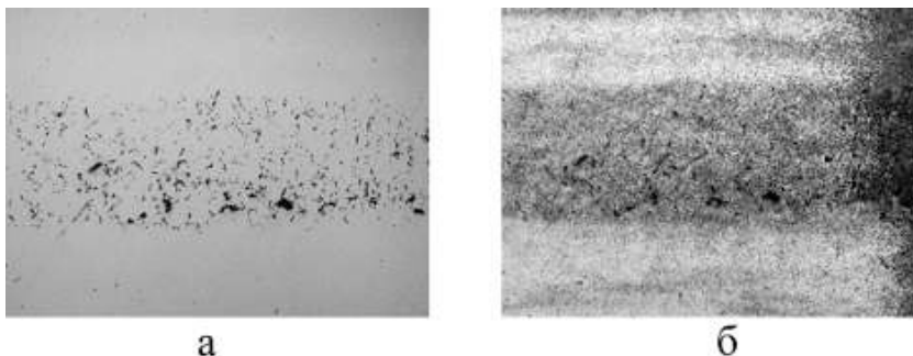
Рис. 5. Микропоры в нетравленых (а) и травленых (б) шлифахподшипниковой стали, \times 100
