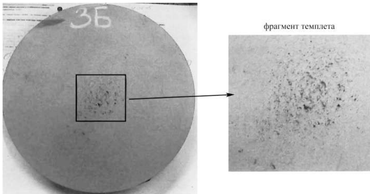
Рис. 4. Макроструктура прутка с микропорами
