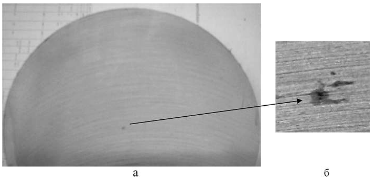
Рис. 3. Макроструктура поковки (а) и фрагмент темплета этой поковки (б) с осевой пористостью слитка, не заварившейся при деформации
