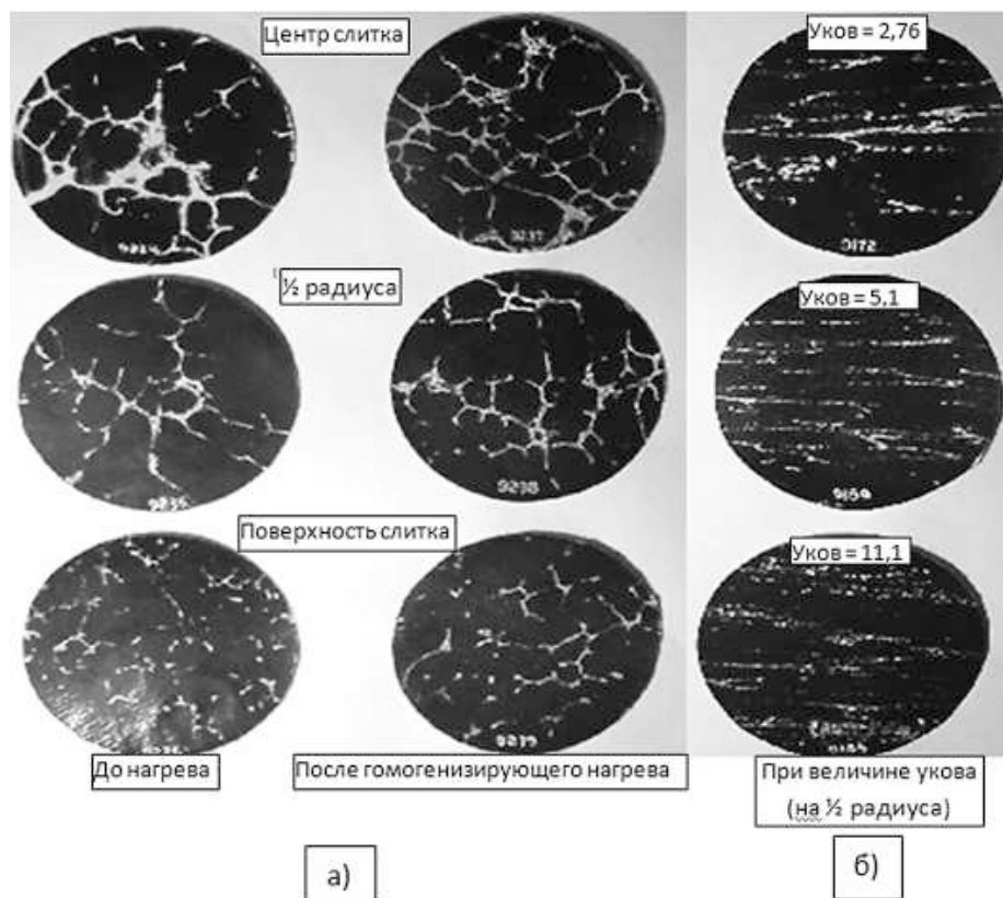
Рис.1. Микроструктура слитка (а) и поковки (б) из стали ЭИ347-III
